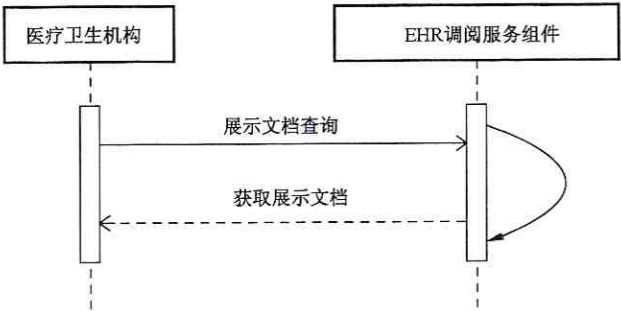
图 85 调阅展示服务调用时序图
