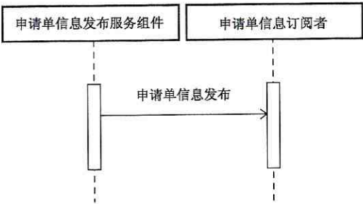
图 39 申请单信息发布服务时序图
