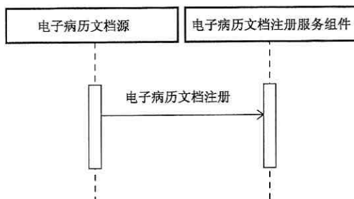
图 61 电子病历文档注册服务时序图
