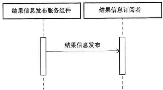
图 57 结果信息发布服务时序图
