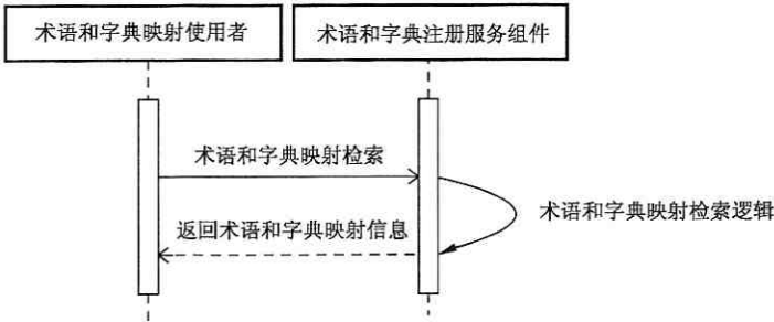
图 17 术语和字典映射服务时序图
