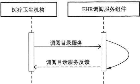
图 87 调阅目录服务调用时序图
