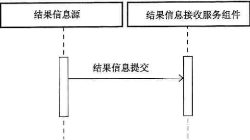
图 51 结果信息接收服务时序图
