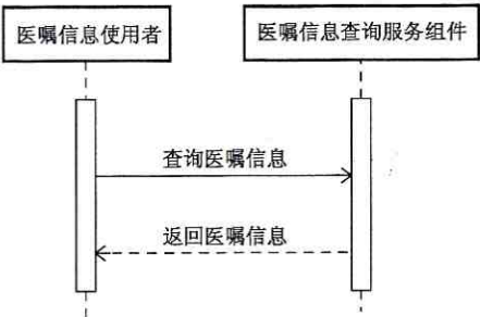
图 33 医嘱信息查询服务时序图
