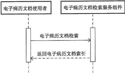
图 63 电子病历文档检索服务时序图
