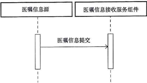
图 27 医嘱信息接收服务时序图
