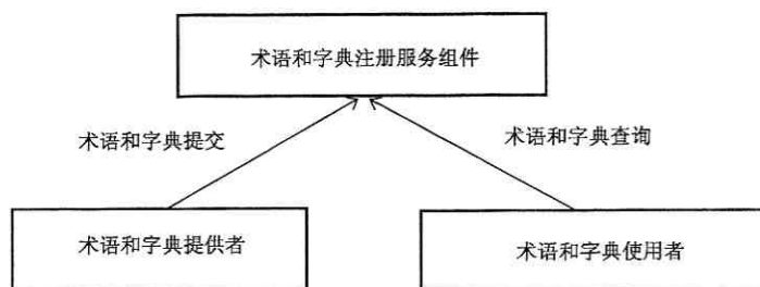
图 14 术语和字典注册角色交易图
