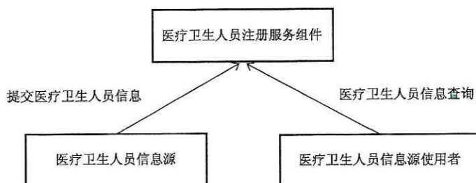
图 10 医疗卫生人员注册角色交易图
