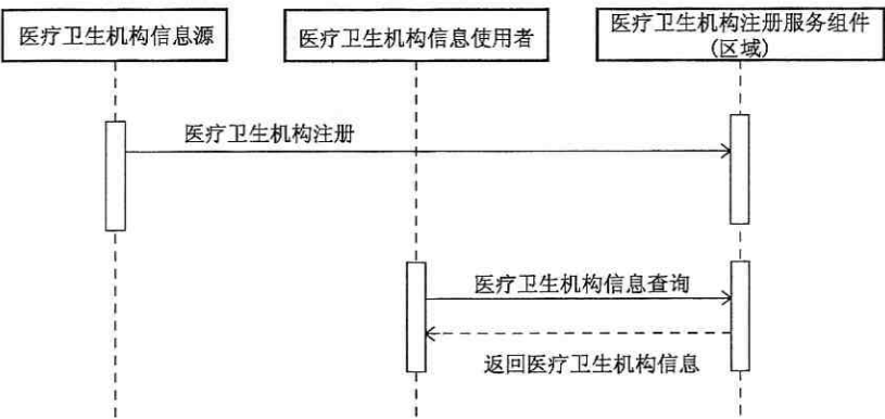
图 77 医疗卫生机构注册服务调用时序图
