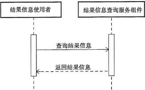
图 55 结果信息查询服务交易时序图
