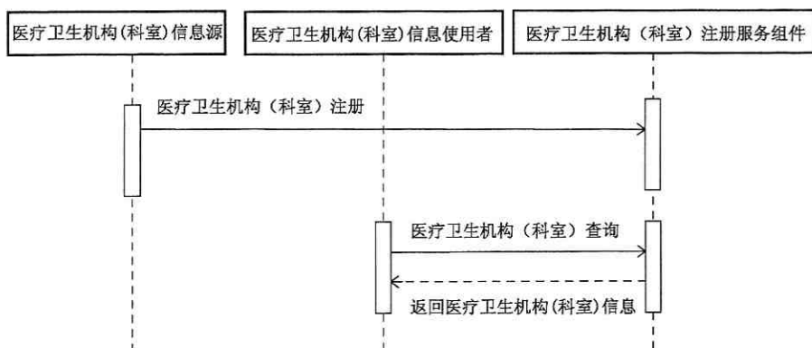
图 13 医疗卫生机构(科室)注册服务时序图
