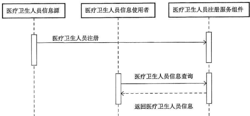
图 11 医疗人员注册服务时序图
