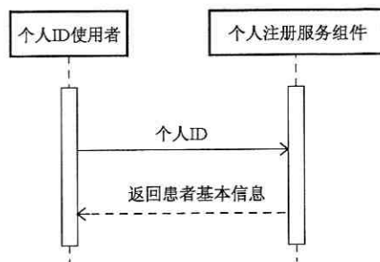
图 9 个人基本信息查询服务时序图
