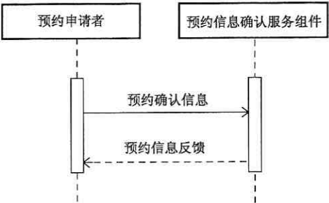
图 47 预约信息确认服务时序图
