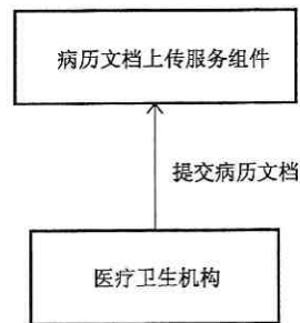
图 90 病历文档上传服务调用角色交易图
