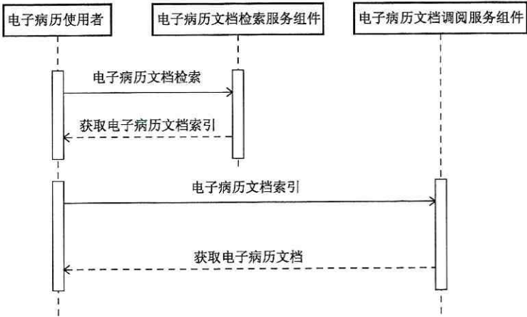
图 67 电子病历文档调阅服务时序图
