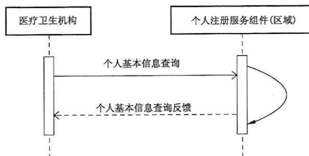
图 73 个人基本信息查询服务调用时序图
