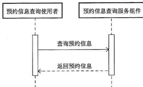
图 49 预约信息查询服务时序图
