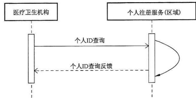
图 71 个人 ID 查询服务调用时序图
