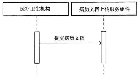
图 91 病历文档上传服务调用时序图
