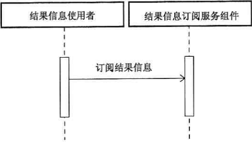
图 59 结果信息订阅服务时序图
