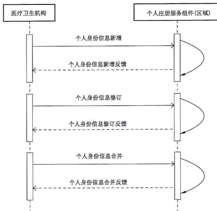
图 69 个人注册服务调用时序图
