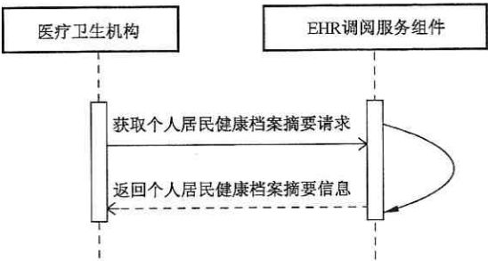
图 89 摘要调阅服务调用时序图
