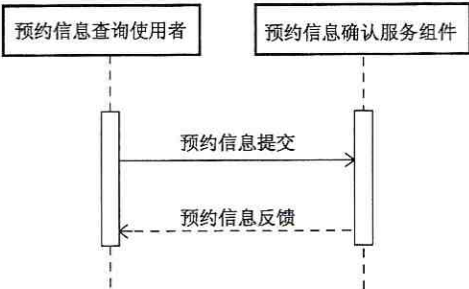
图 48 预约信息查询服务角色交易图
