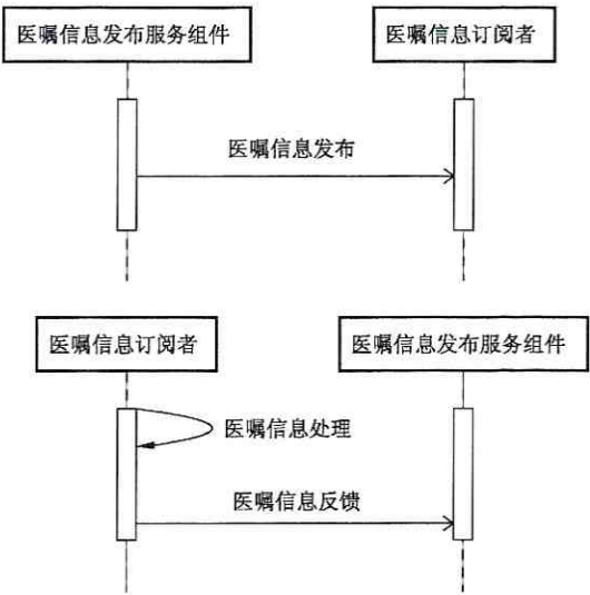
图 31 医嘱信息发布服务时序图
