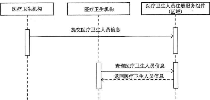
图 75 医疗卫生机构注册服务调用时序图
