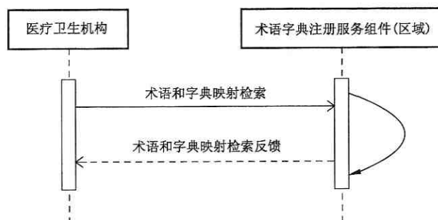
图 81 术语和字典映射服务调用时序图
