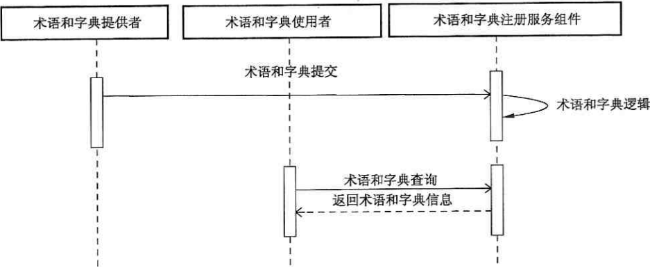
图 15 术语和字典注册服务时序图
