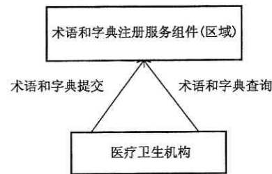
图 78 医疗卫生和术语字典注册服务调用角色交易图
