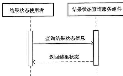
图 53 结果状态查询服务时序图
