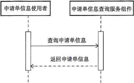
图 41 申请单信息查询服务时序图
