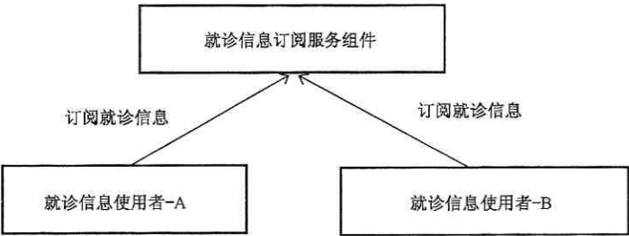
图 20 就诊信息订阅角色交易图
