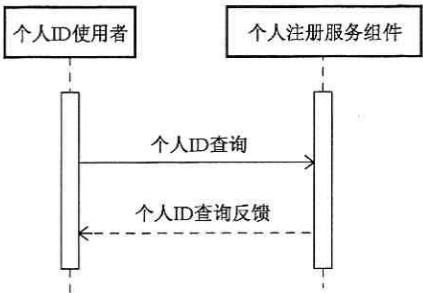
图 7 个人 ID 查询服务时序图
