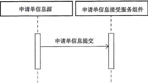
图 35 申请单信息接收服务时序图
