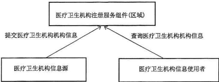
图 76 医疗卫生机构注册服务调用角色交易图
