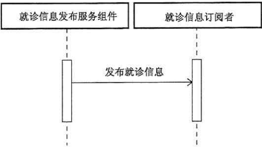
图 23 就诊信息发布服务时序图
