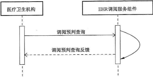
图 83 调阅预判服务调用时序图
