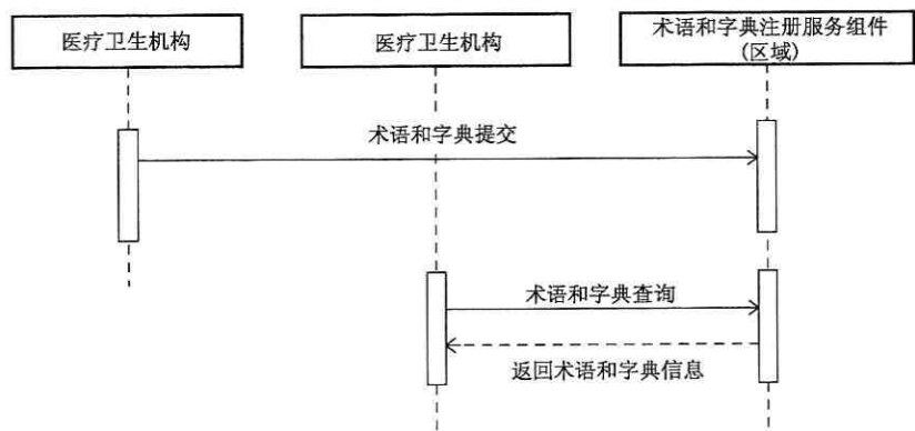
图 79 医疗卫生术语和字典注册服务调用时序图
