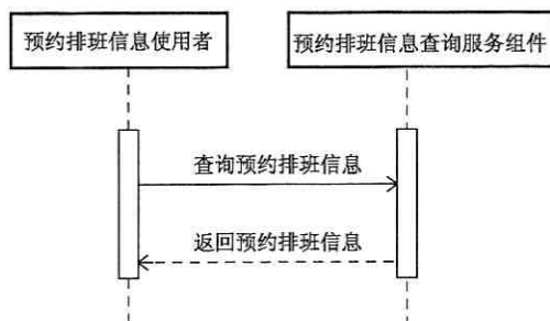
图 45 预约排班信息查询服务交易时序图
