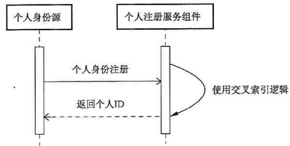
图 5 个人身份注册服务时序图
